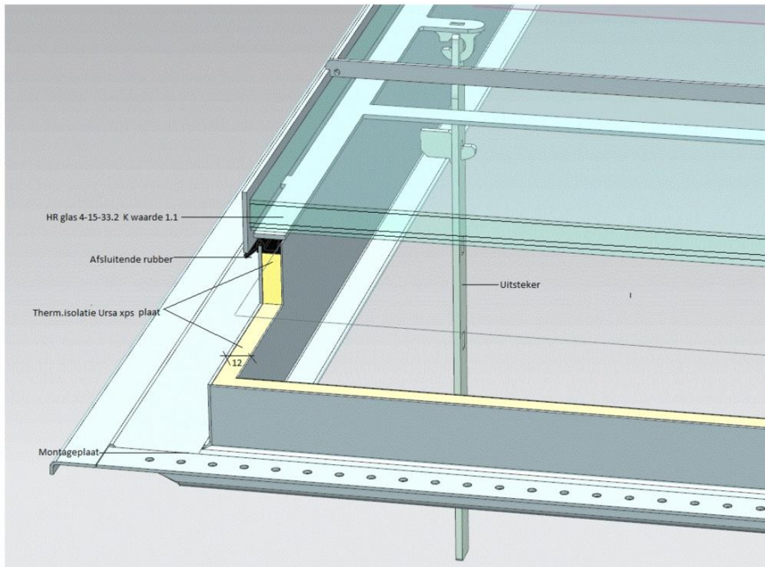
Sparing maat met boog H 642 x R 114 x B 594 (zonder speling)
