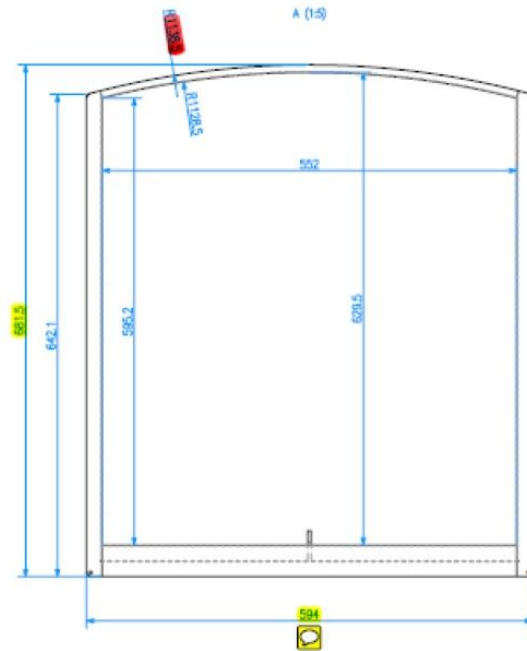
Sparing maat met boog H 642 x R 114 x B 594 (zonder speling)
