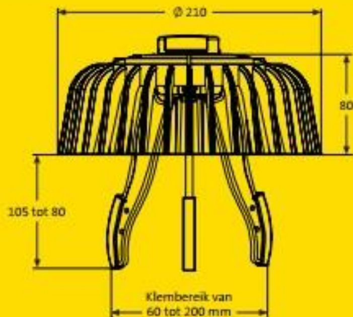
Technische tekening
