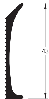
Artikelnummer 151600 (schaal 1:1)
