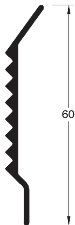
Artikelnummer 151590 (schaal 1:1)
